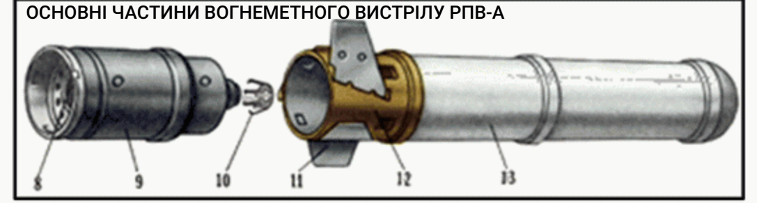
ОСНОВНІ ЧАСТИНИ ВОГНЕМЕТНОГО ВИСТРІЛУ РПВ-А
